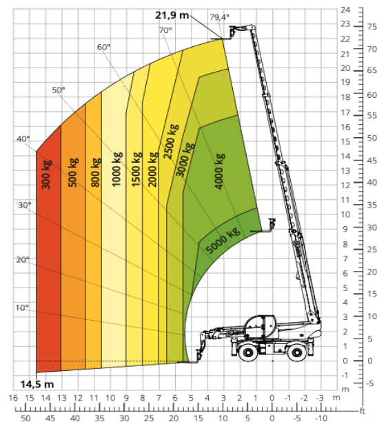
Abaque de charge FRONTAL SUR PNEUS ATT - 03 - 001
