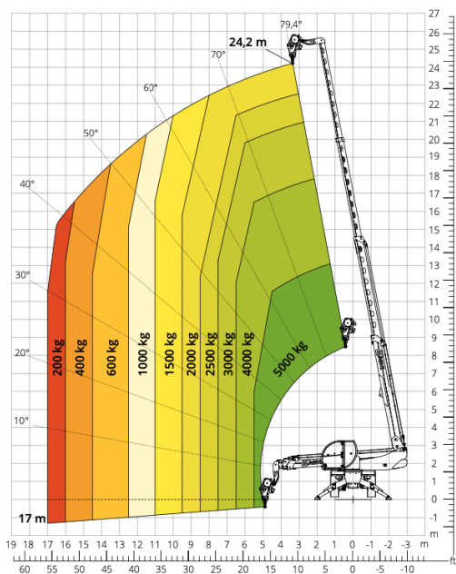
Abaque de charge avec TREUIL 5 000 kg ATT - 02 - 019
