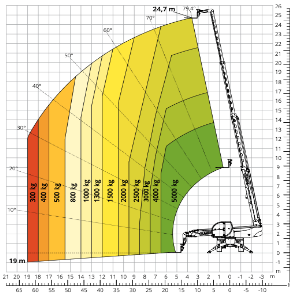
Abaque de charge avec STABILISATEURS DÉPLOYÉS 360° ATT - 03 - 001
